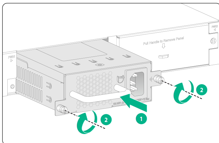
图2-23 安装电源模块示意图
