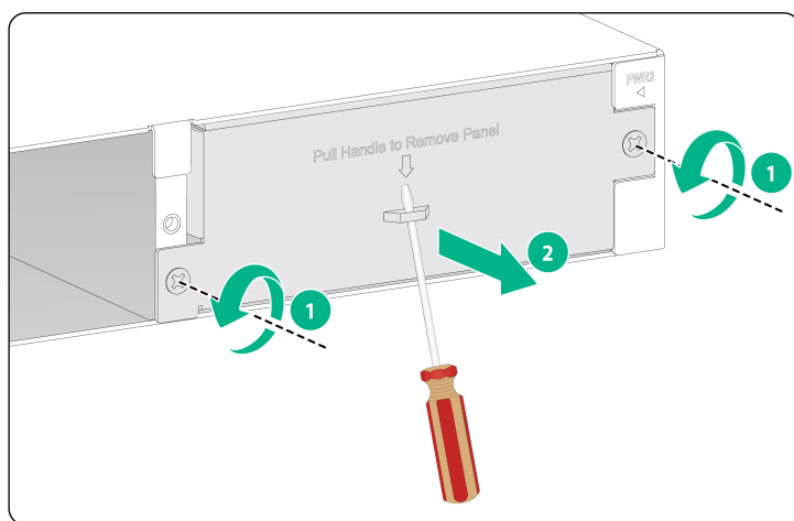
图2-24 拆卸电源假面板示意图
