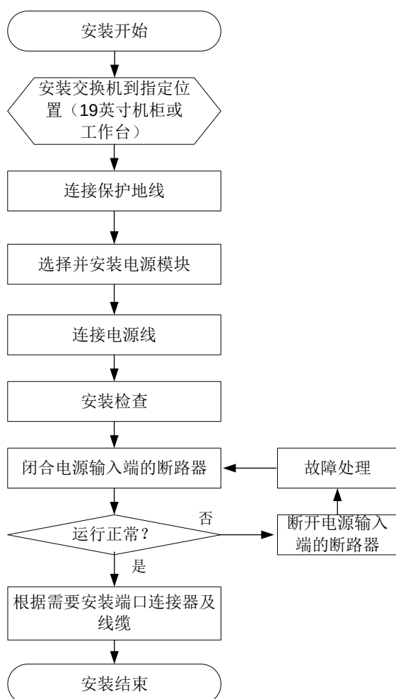
图2-1 交换机硬件安装流程
