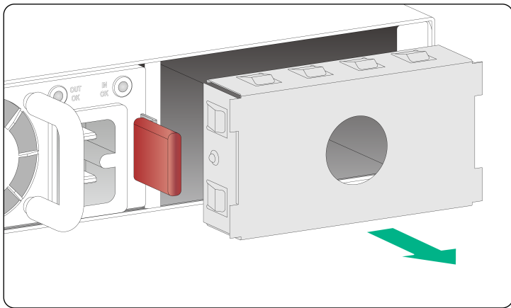
图2-21 电源假面板拆卸示意图
