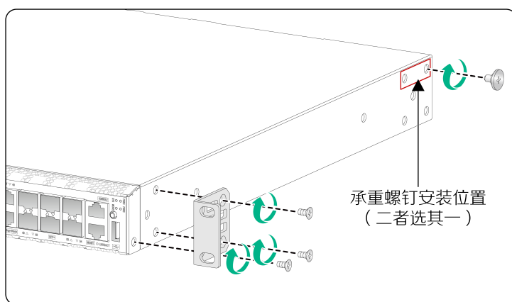
图2-9 安装前挂耳和承重螺钉到设备的示意图（端口侧）
