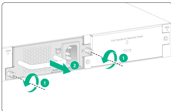
图2-25 拆卸电源模块示意图
