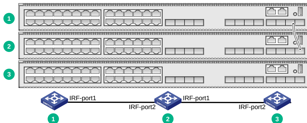
图4-2 IRF 链型连接方式及对应的拓扑示意图
