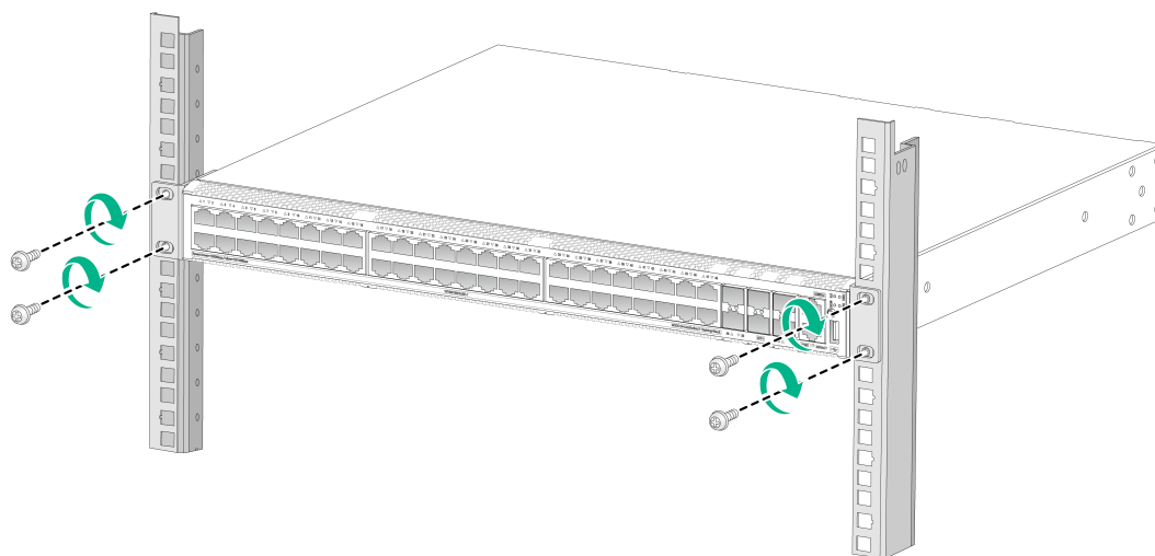
图2-8 安装交换机到机柜示意图
