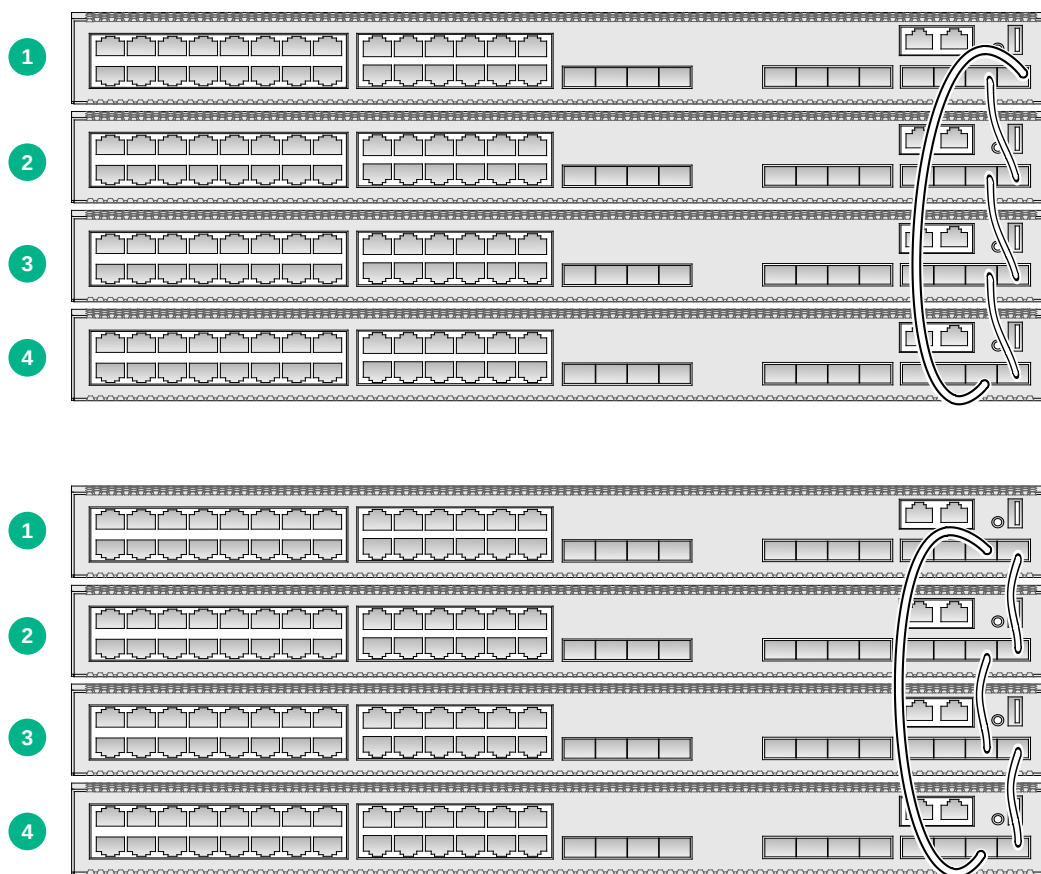
图4-4 集中式放置环形连接示意图
