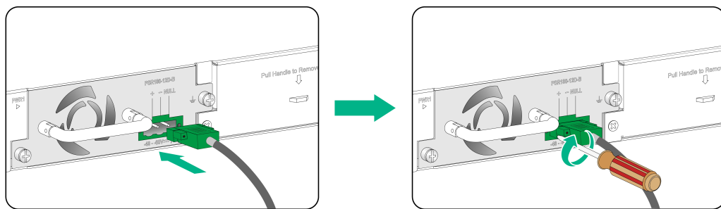
图2-28 连接 PSR180-12D-B 电源线示意图
