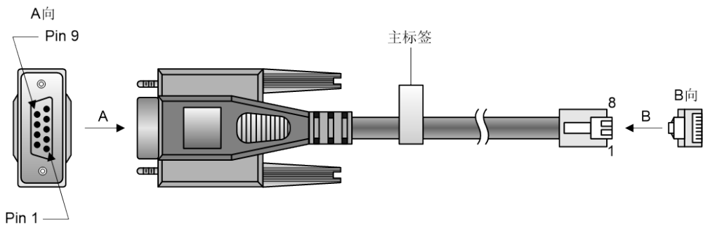
图3-2 DB9-to-RJ45 Console 口电缆示意图
