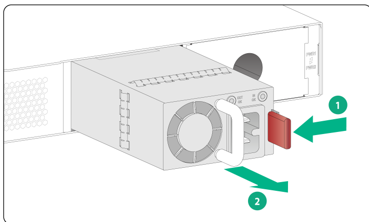
图2-22 拆卸电源模块
