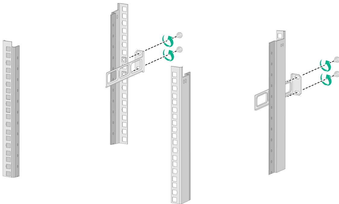
图2-11 正向安装后挂耳到机柜方孔条示意图
