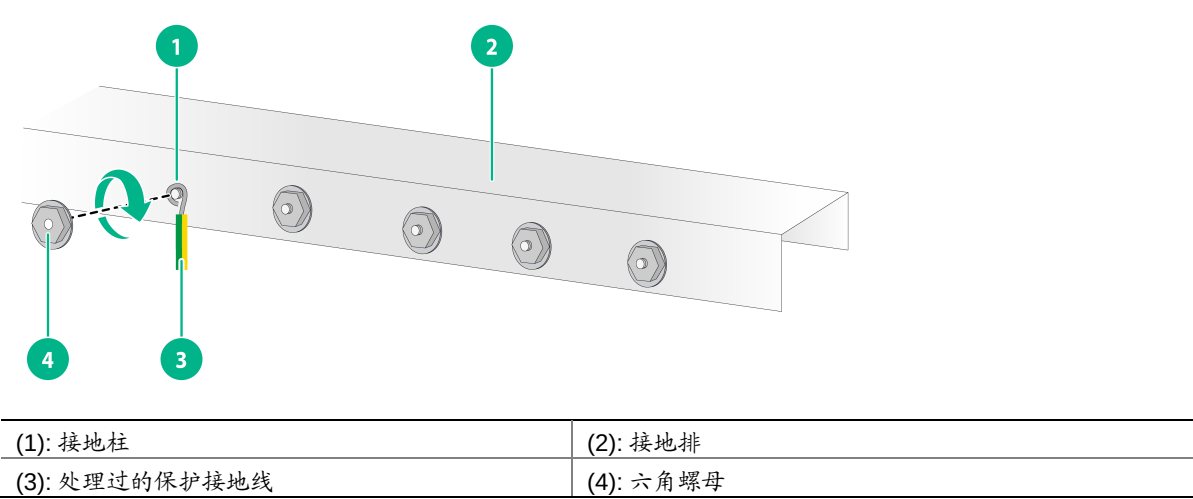
图2-16 连接保护接地线到接地排
