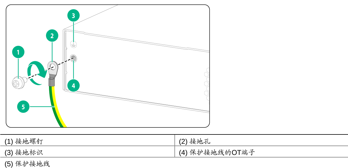
图2-15 连接保护地接线到交换机的接地孔
