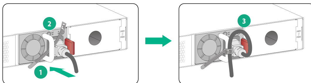
图2-26 PSR600-54A-B 电源线连接示意图
