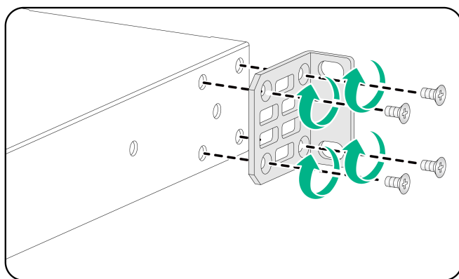
图2-7 安装前挂耳到设备电源侧的示意图
