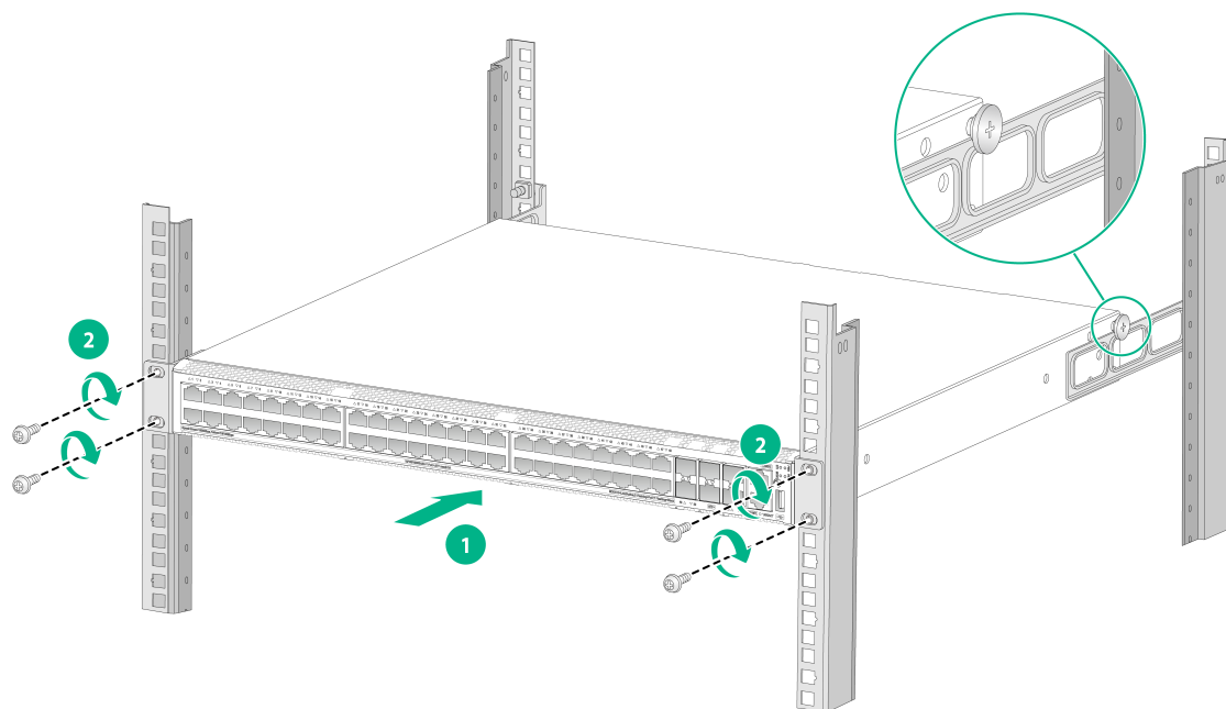
图2-13 安装交换机到机柜示意图（后挂耳正向安装到机柜方孔条）
