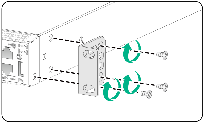
图2-6 安装前挂耳到设备端口侧的示意图
