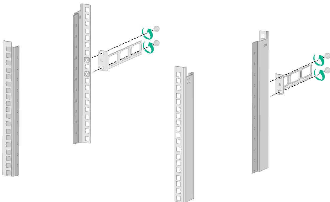
图2-12 反向安装后挂耳到机柜方孔条示意图
