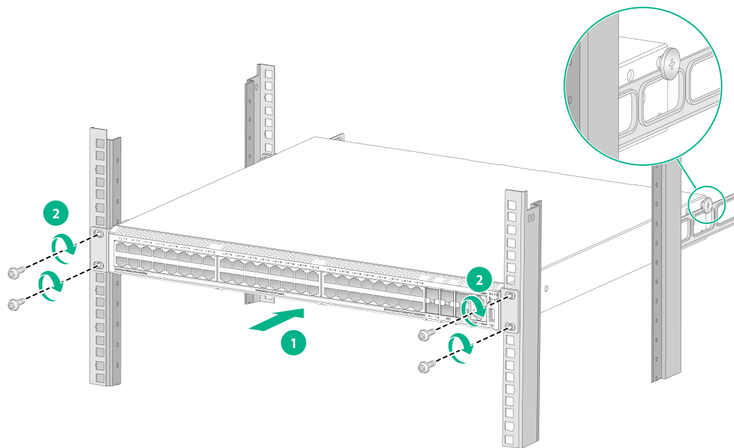
图2-14 安装交换机到机柜示意图（后挂耳反向安装到机柜方孔条）
