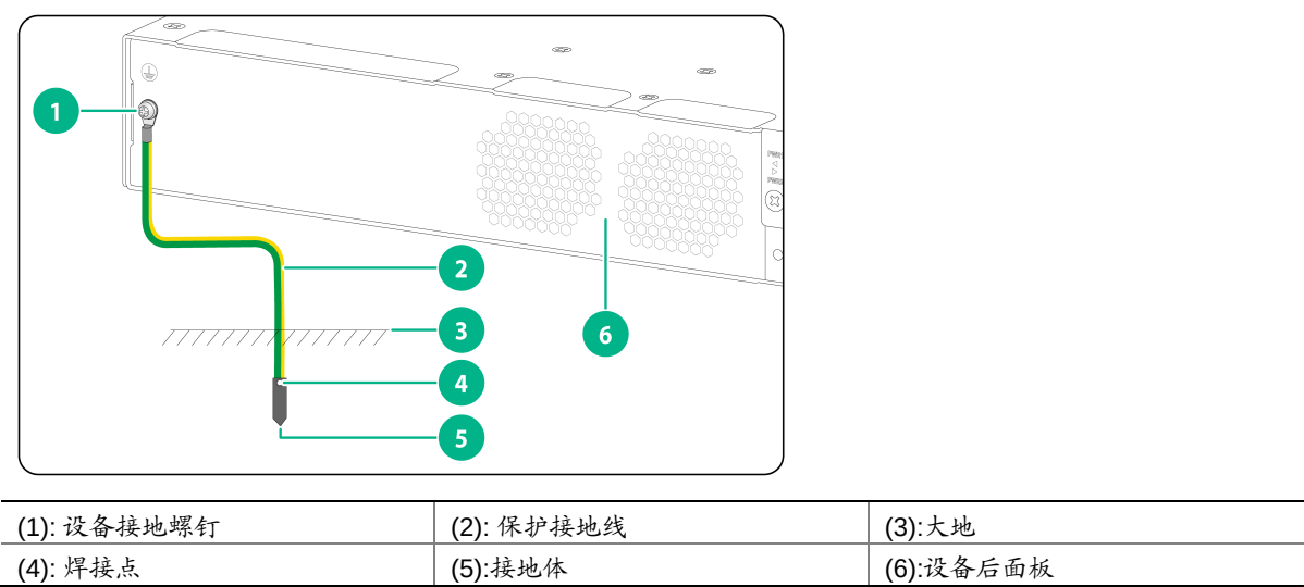
图2-17 机房附近允许埋设接地体时接地安装示意图
