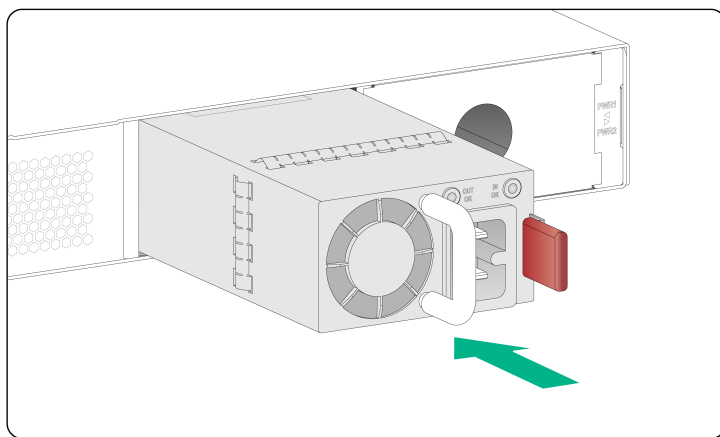
图2-20 电源模块安装示意图
