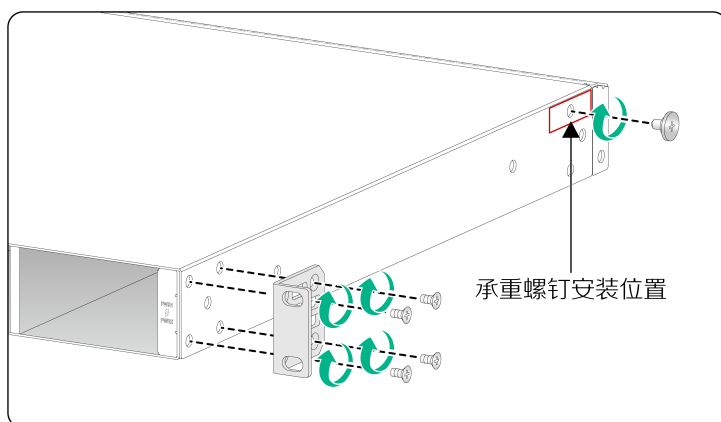
图2-10 安装前挂耳和承重螺钉到设备的示意图（电源侧）
