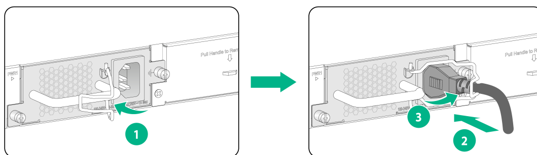
图2-27 连接 CA-70A12 电源线示意图
